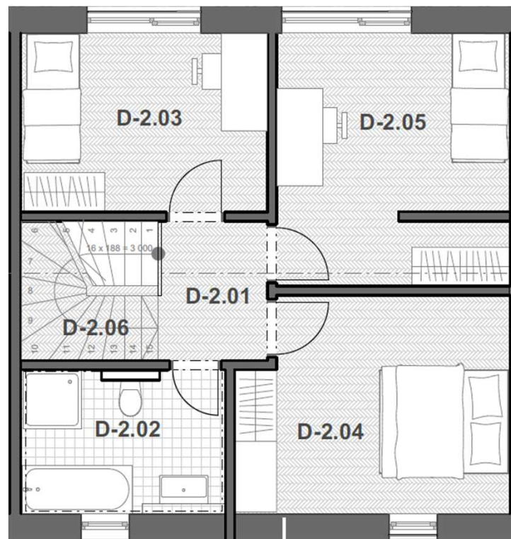
PŮDORYS 2.NP
