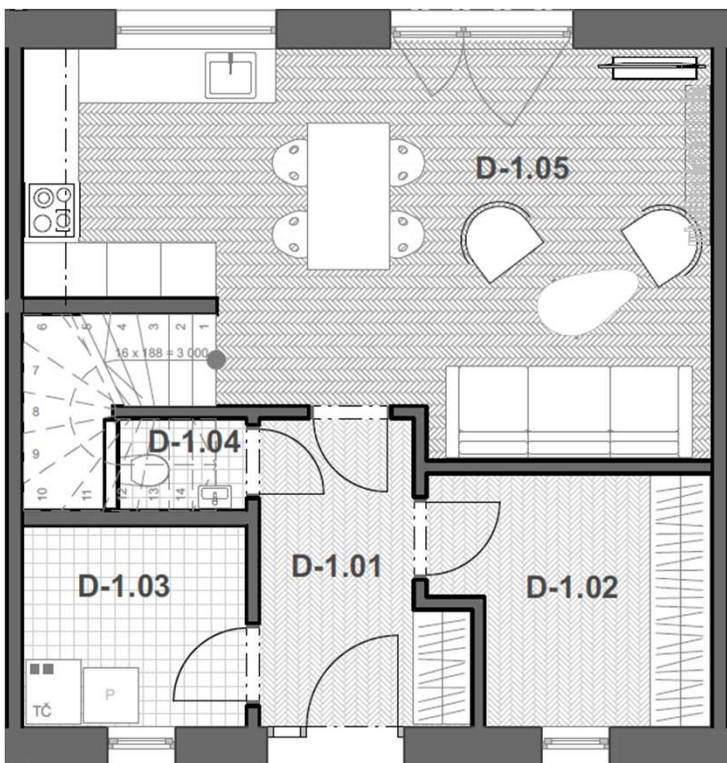
PŮDORYS 1.NP
