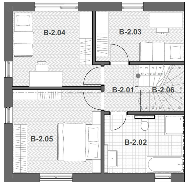
PŮDORYS 2.NP
