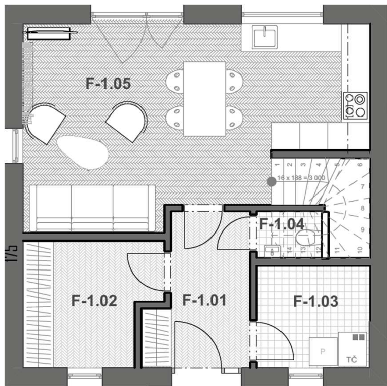
PŮDORYS 1.NP
