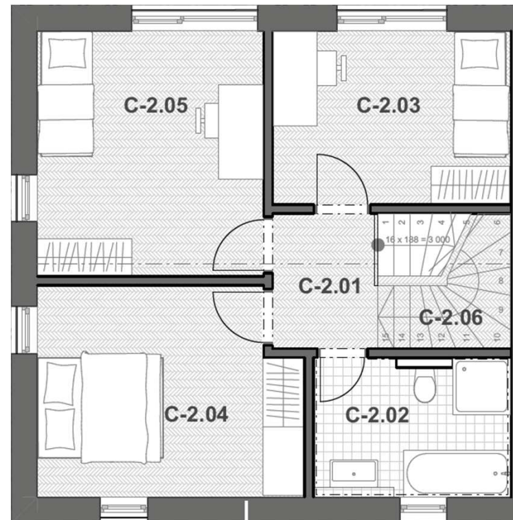
PŮDORYS 2.NP
