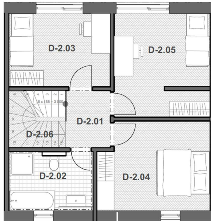
PŮDORYS 2.NP
