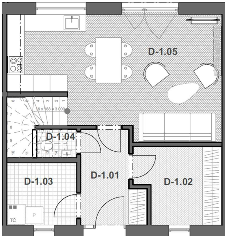
PŮDORYS 1.NP
