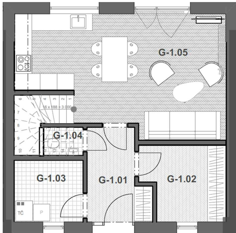
PŮDORYS 1.NP
