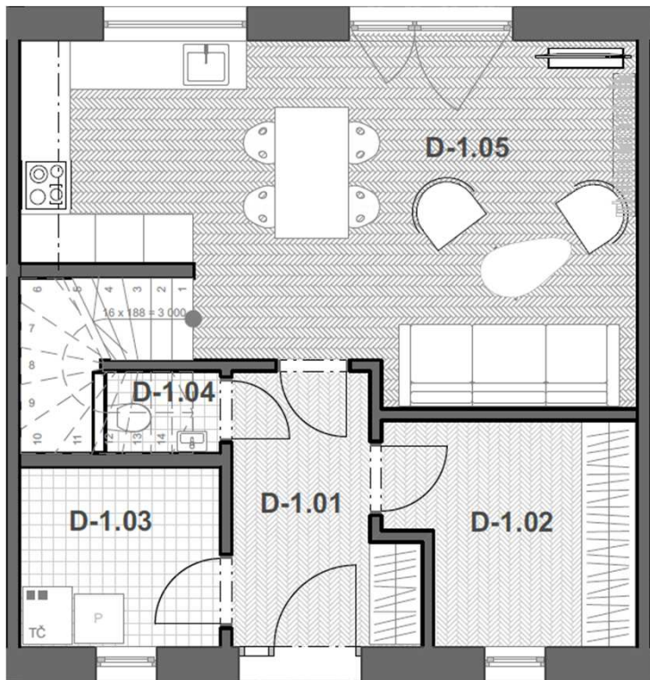
PŮDORYS 1.NP
